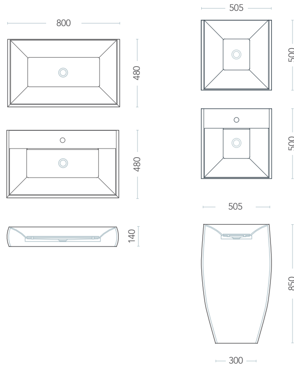
Duna 1/2 lavabo da appoggio countertop washbasin Aufsatzbecken
